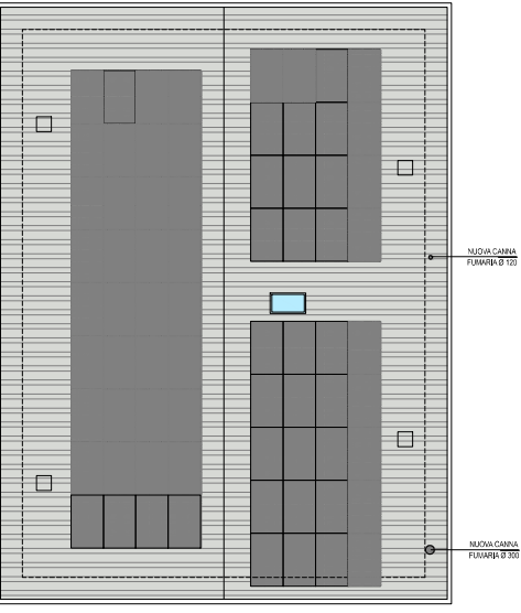
PIANTA COPERTURA
